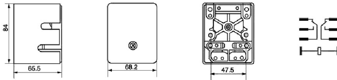
JQX-62F 2Z
